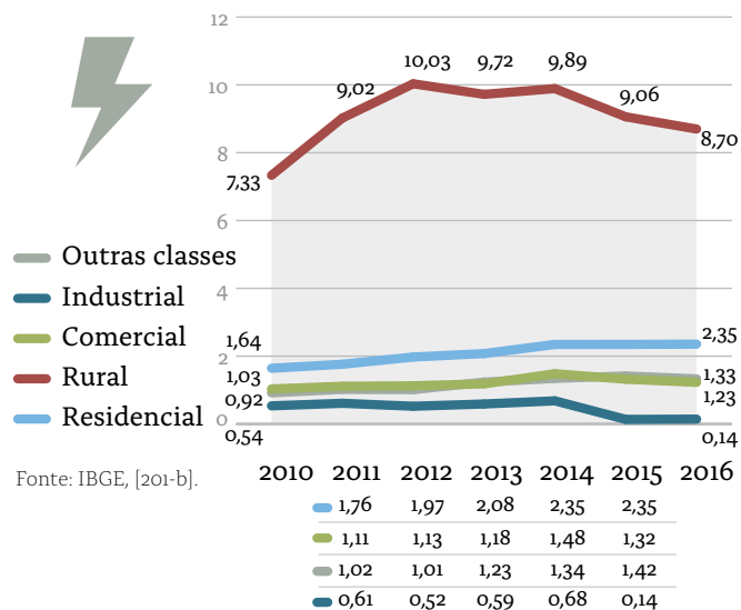
Gr fico 25: Consumo total de energia do munic pio, por setor, em GWh, de 2010 a 2016
