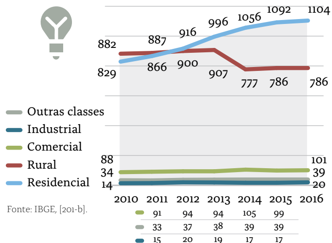
Gr fico 26: N mero total de consumidores do munic pio, por setor, de 2010 a 2016
