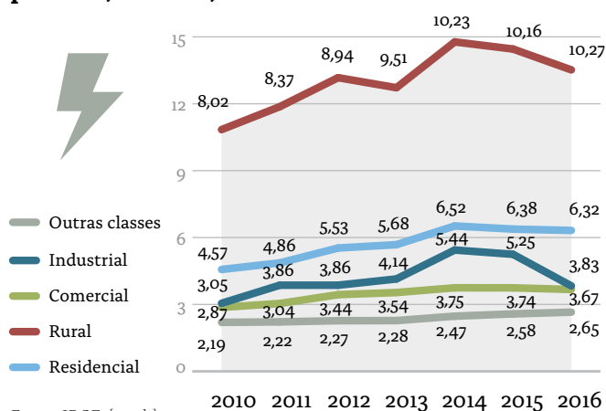
Gr fico 25: Consumo total de energia do munic pio, por setor, em GWh, de 2010 a 2016
